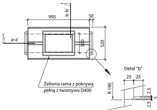
Widok "a"="b" II-0-CS - pióro/pióro
