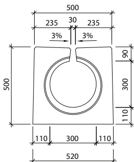
Widok "a"="b" II-0-CS - pióro/pióro
