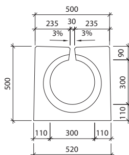
Widok "a" II-0-C0 - wpust
