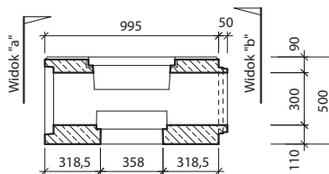
Przekrój: a-a' II-0-V0
