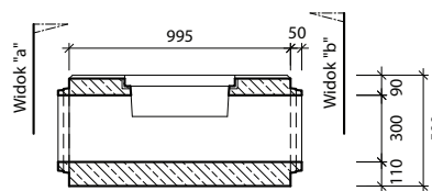
Przekrój: a-a'
