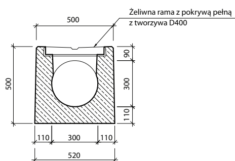
Przekrój: b-b'
